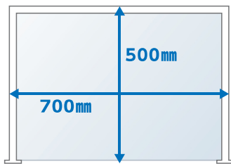
型番: FFP-HSS-75 W700×H500×D75
