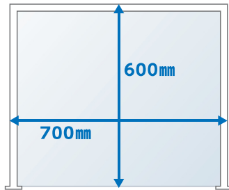
型番: FFP-HSS-76 W700×H600×D75
